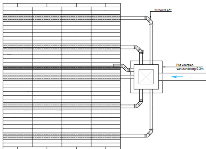
Elk Rockflow-kanaal moet vanuit een inspectieput middels Ø125 leiding met maximaal 45° bochten bereikbaar zijn in het basisonwerp zit een kanaal h.o.h. 1,20m
