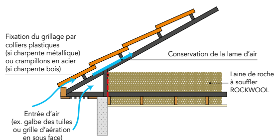
Figure 3 : Schéma de principe de la mise en œuvre du grillage de confinement sur une charpente industrielle métallique « petit entrain »
