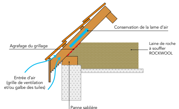
Figure 1 : Schéma de principe de la mise en œuvre du grillage de confinement sur une charpente traditionnelle
