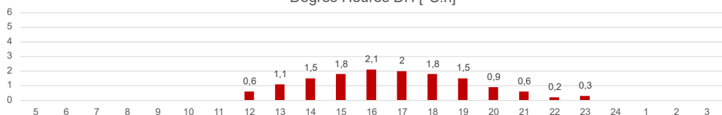
Degrès Heures DH [°C.h]
