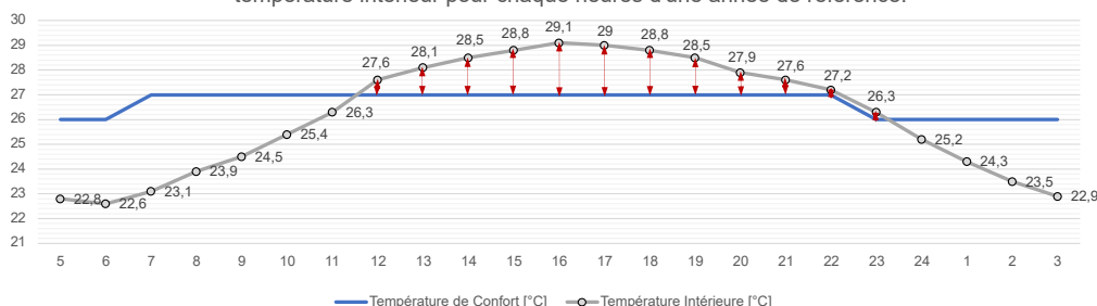
Méthode de calcul des Degrès Heures en fonction de la température de confort et de la température intérieure pour chaque heures d'une année de référence.
