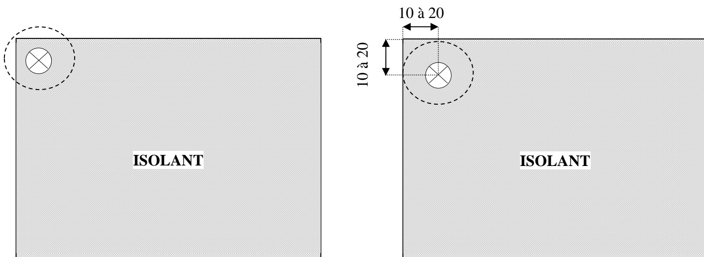
Figure 1 - Position de la fixation mécanique des panneaux
