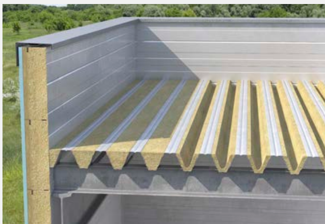
Wypełnienie fałd blachy wkładkami RAW lub welonem szklanym wraz z BLOCZKAMI TRAPEZOWYMI ROCKWOOL.
