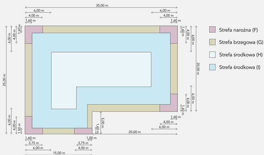
Przykładowy podział stref wiatrowych na dachu płaskiego, zgodnie z: Eurokod 1. Oddziaływania na konstrukcję. Część 1-4: Oddziaływania ogólne. Oddziaływania wiatru.
